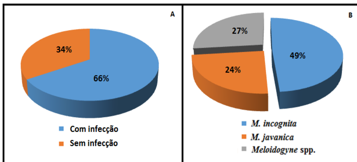
Figura 4 – (A) Percentual de amostras infectadas com nematoides das galhas radiculares. (B) Percentual de Meloidogyne spp. nas amostras infectadas. Amostras oriundas de áreas produtoras de hortaliças da região Sul do Estado de Goiás coletadas no triênio 2013 a 2015.
