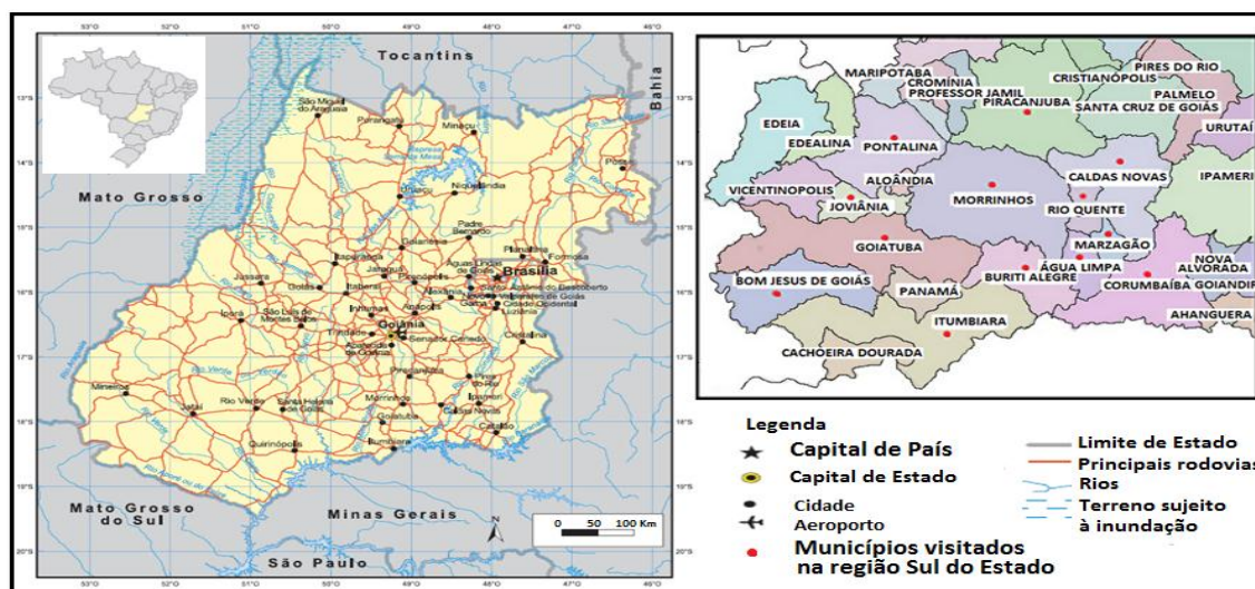
Figura 1 – Mapa de Goiás exibindo a localização dos municípios da região Sul onde foi realizado as coletas de amostras de solo e raízes em áreas de cultivo de hortaliças para análises nematológicas no triênio 2013 a 2015. (IBGE, 2015).
