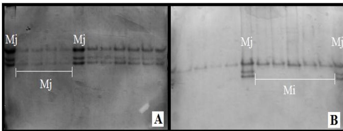
262 263 Figura 5 – Fenótipos de esterase de fêmeas extraídas de duas amostras de raízes de quiabeiro: (A) 264 Meloidogyne javanica - Mj e (B) Meloidogyne incognita - Mi de amostras coletadas na 265 região Sul do Estado de Goiás no triênio de 2013 a 2015. 266
