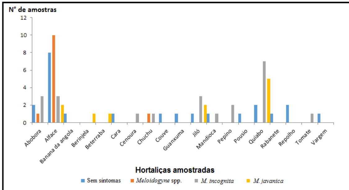
Figura 6 – Quantidade de amostras, infectadas ou não, com as espécies M. incognita e M. javanica e Meloiodogyne spp., coletadas na região Sul do Estado de Goiás no triênio 2013 a 2015.
