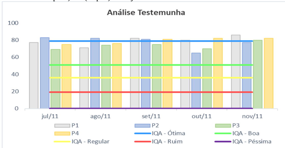
Gráfico 1 - Análise testemunha do IQA nos pontos 1 (Ribeirão Cima), 2 (Araguaia), 3 (Três Capões) e 4 (Capão) entre julho de 2011 e novembro de 2011
