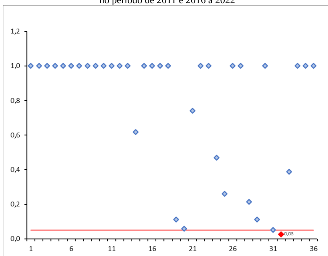
Gráfico 7 - Diferença estatística a partir do Teste de Kruskal-Wallis (Teste de Dunn) do IQA no período de 2011 e 2016 a 2022
