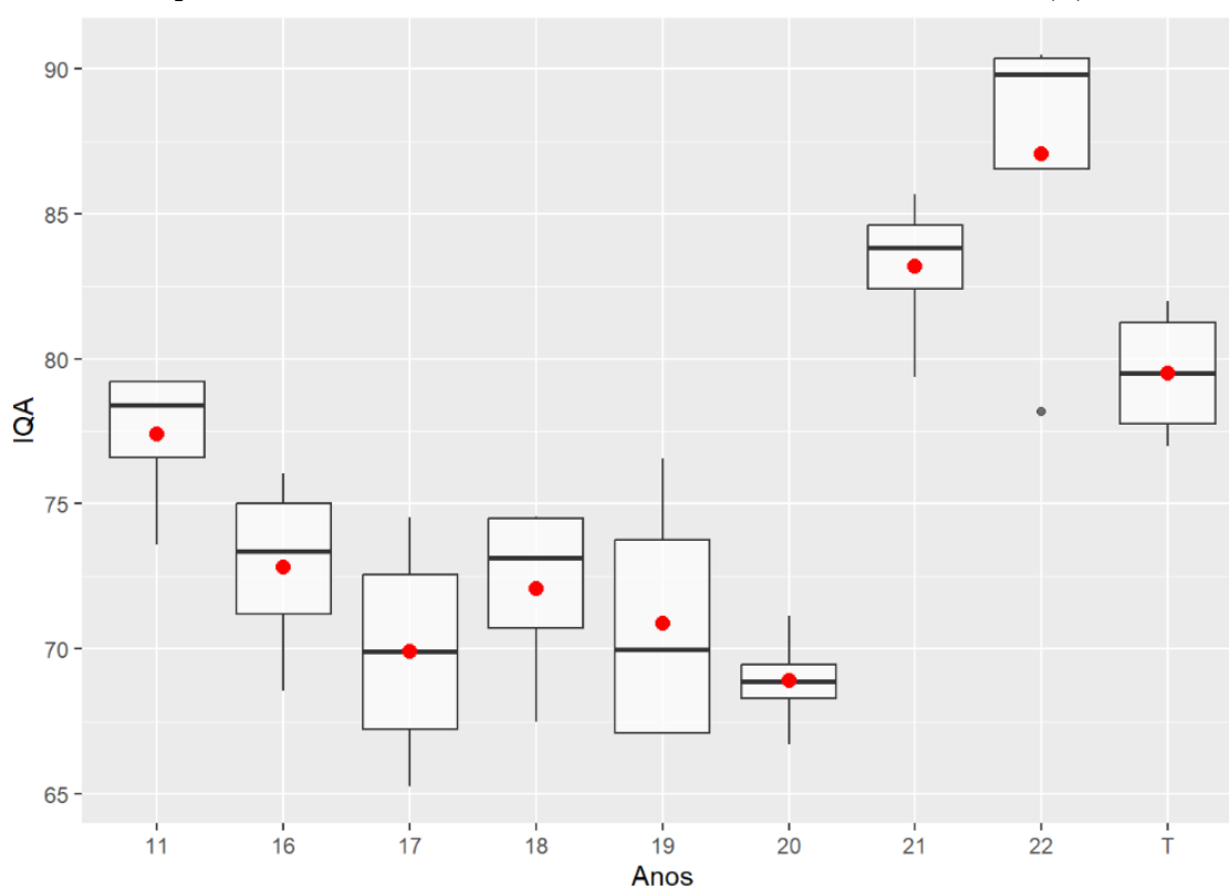
Gráfico 6 - Boxplot do índice histórico da qualidade da água (IQA) dos pontos 1 (Ribeirão de Cima), 2 (Rio Araguaia), 3 (Córrego Três Capões) e 4 (Córrego Capão) considerando o período de 2011, maio de 2016 a maio de 2021 e testemunha (T)
