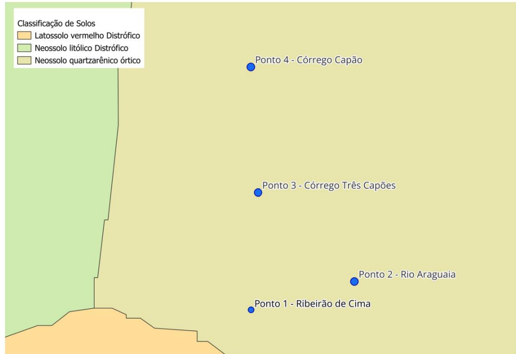
Figura 1 - Classificação de solos para o Município de Alto Taquari
