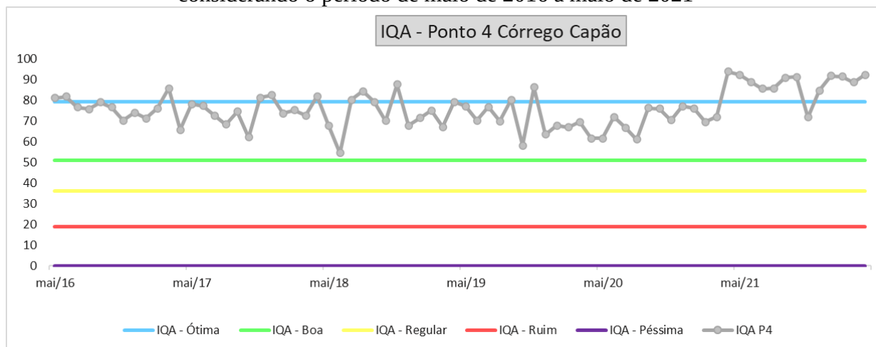
Gráfico 5 - Índice histórico da qualidade da água (IQA) do ponto 4 (Córrego Capão) considerando o período de maio de 2016 a maio de 2021
