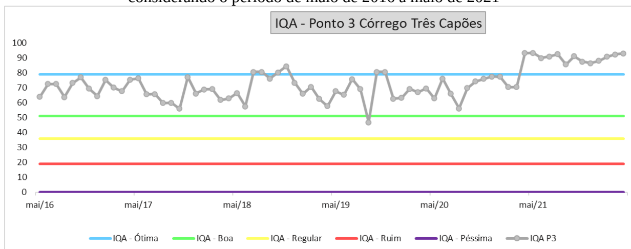
Gráfico 4 - Índice histórico da qualidade da água (IQA) do ponto 3 (Córrego Três Capões) considerando o período de maio de 2016 a maio de 2021
