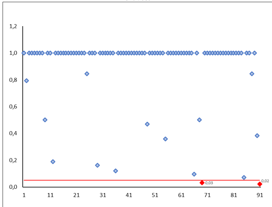
Gráfico 8 - Diferença estatística a partir do Teste de Kruskal-Wallis (Teste de Dunn) do IQA no período de 2011 e 2016 a 2022 a partir da comparação entre a estação seca e estação chuvosa
