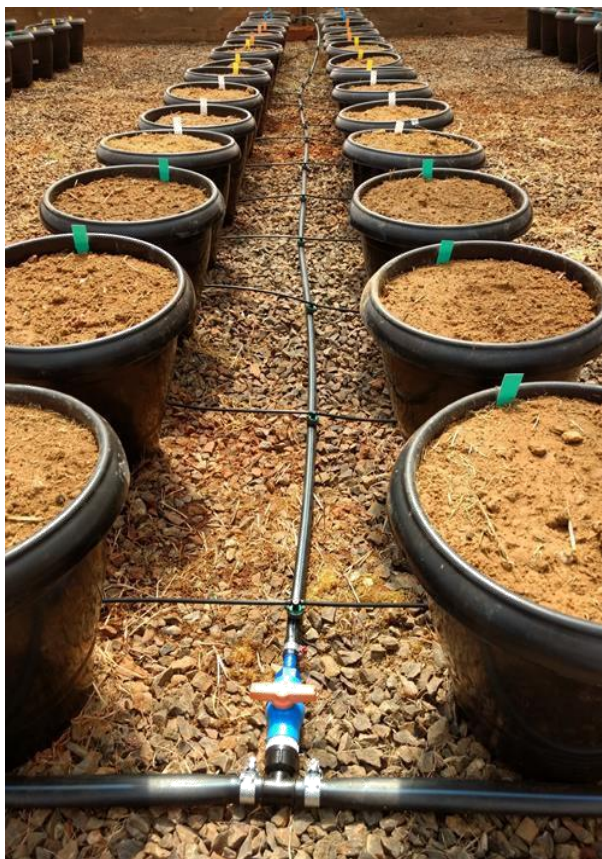
Figura 5. Linha lateral de sistema por gotejamento para cultivo de tomateiro em linhas duplas.
