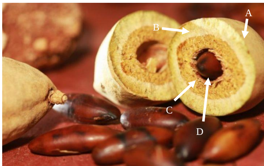
Figura 2- Fruto do baru integral e suas partes: (A) Epicarpo, (B) Mesocarpo, (C) Endocarpo e (D) amêndoa
