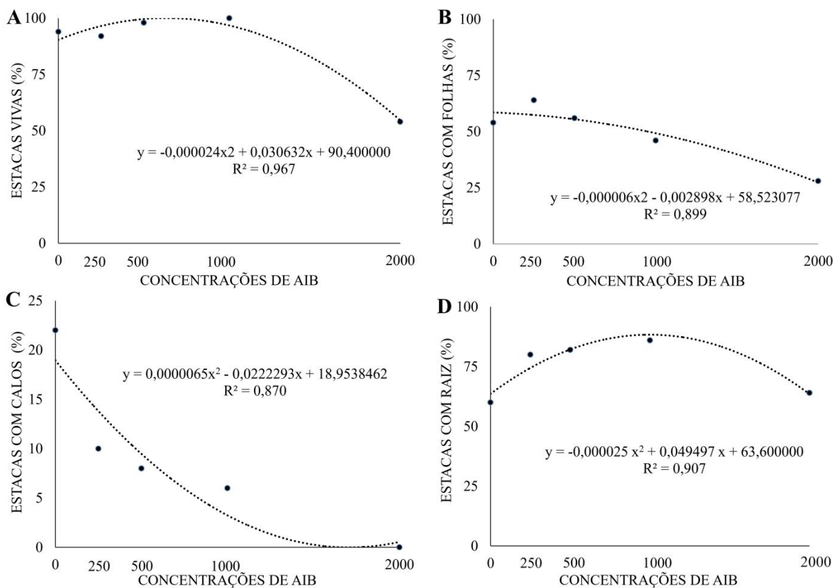
Figura 2. (A) Estacas vivas; (B) Estacas com folhas; (C) Estacas com calo; e (D) Estacas com raiz de maracujá do Cerrado sob a aplicação de diferentes concentrações de AIB. Ceres, GO. 2019.
