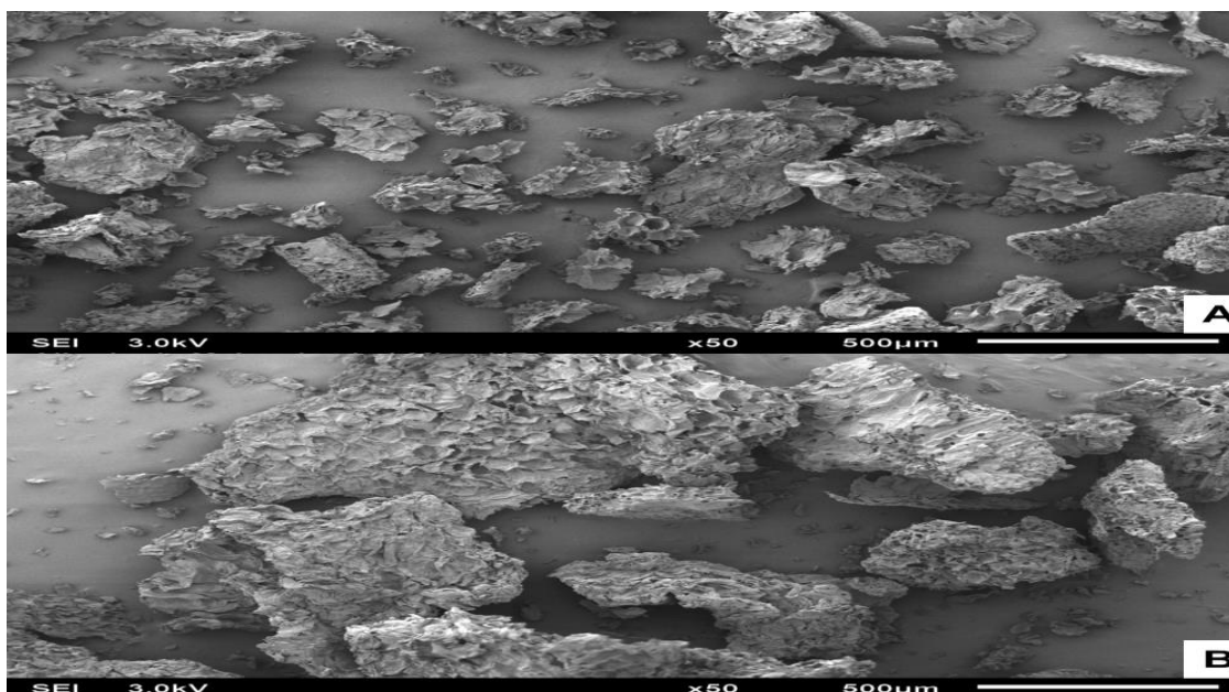
Figura 2. Micrografias eletrônicas por varredura das farinhas da casca (FCM) em (A) e entrecasca (FEM) em (B) de melancia var. Crimson Sweet Extra .
