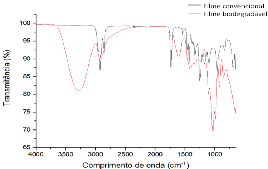
Figura 3. Espectros de absorção na região média do infravermelho entre 4000-650 \text{cm}^{-1} do filme convencional (PVC) e biofilme de Citrullus lanatus .
